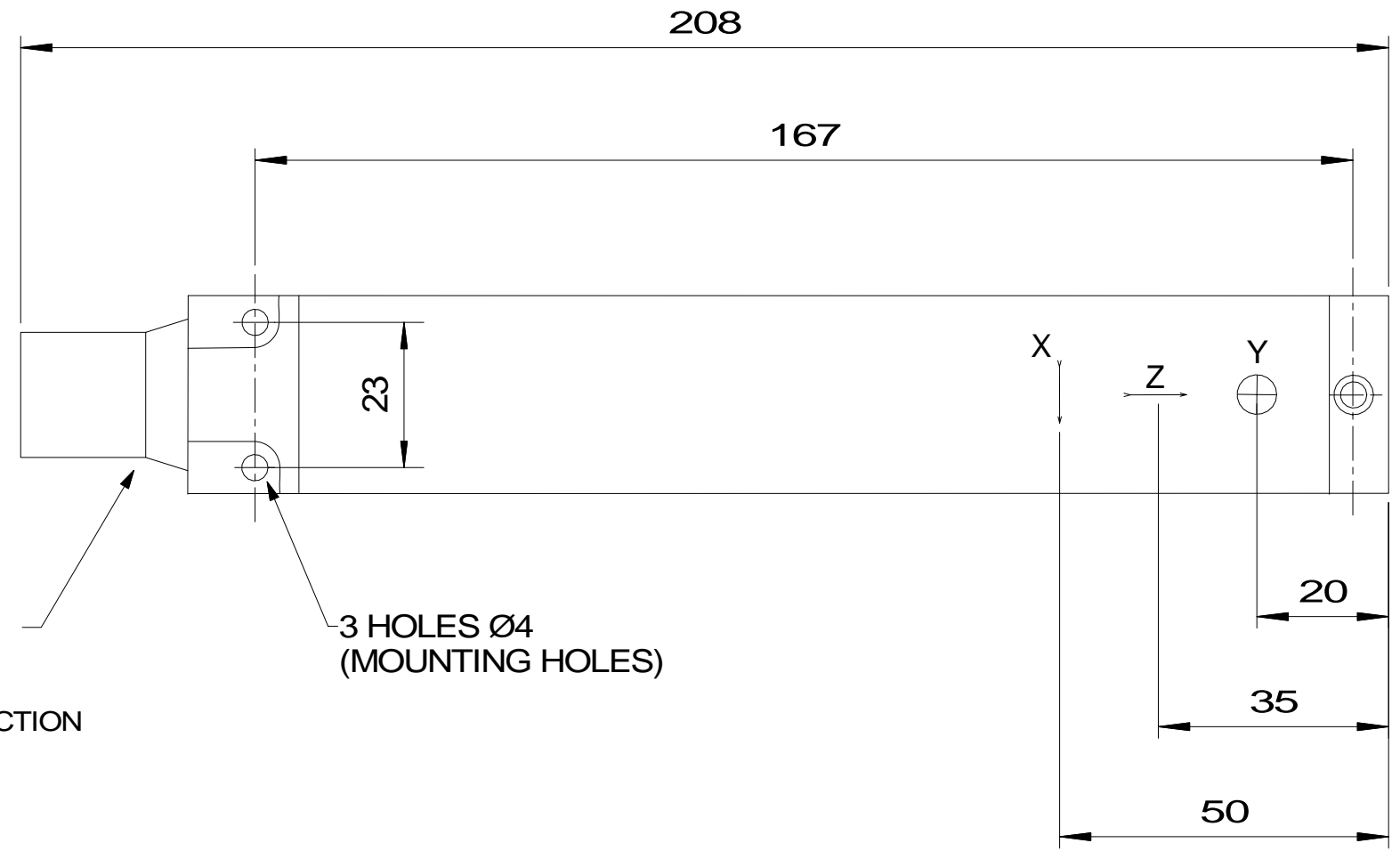
BULKHEAD IE-XSJ-7-BCR
